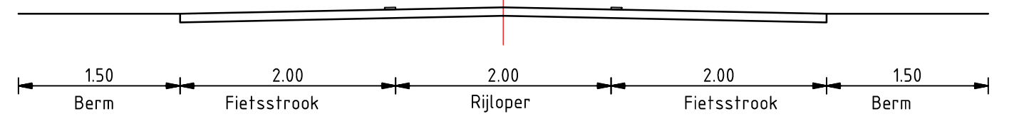
Principeprofiel Bubeko 60 km/h Schaal 1:50
