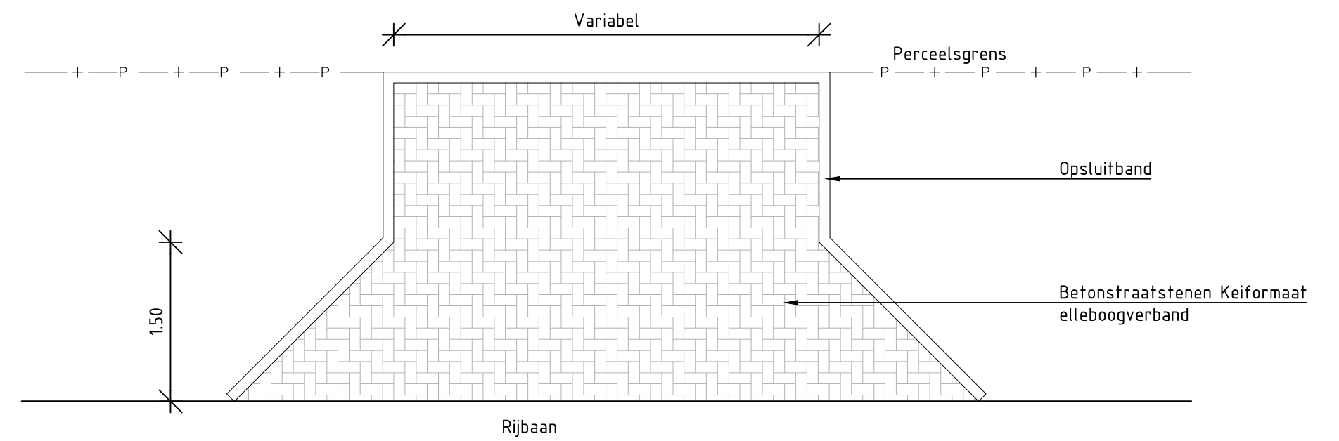
Principe inrit Schaal 1:50
